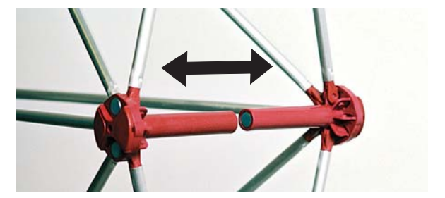
Ved oppmontering av aluminiumsstrukturen låses de magnetiske tverstagene automatisk. Alle avlås samtidig automatisk, ved nedmontering !
