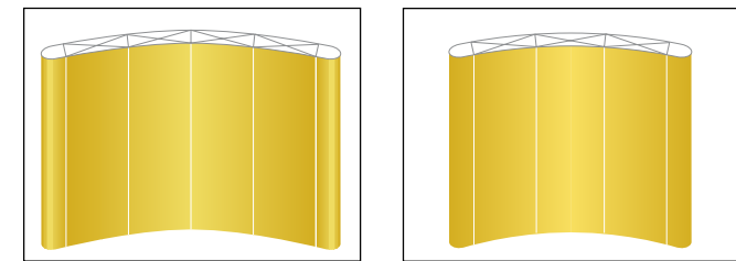
MP1 - 4x3, varenr. 82204 2875 (b) x 2255 (h) x 840 (d) mm MP2 - 4x3, varenr. 82214 3150 (b) x 2225 (h) x 960 (d) mm
